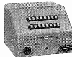
514
