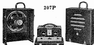
207P
