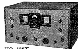
HQ 129X
